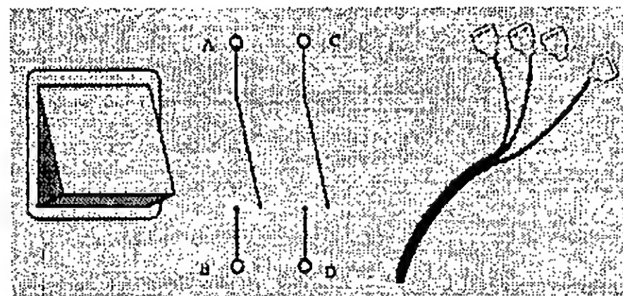
Figura 45 - chave liga-desliga e seu diagrama elétrico
